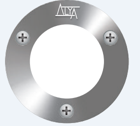
Dairesel Bıçak Tutacağı/Circular Knife Holder 50x30mm, 3xVida/Screw, 1xMil Sabitleme Deliği/Fixing Hole, Paslanmaz/Stainless
